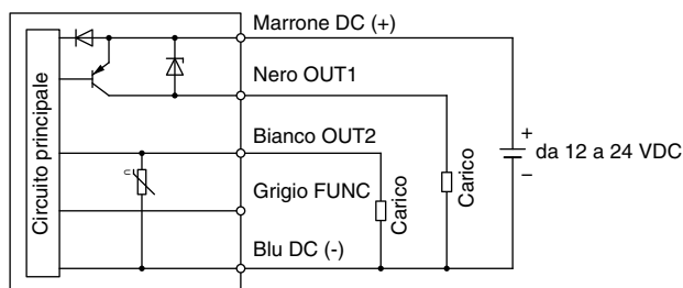
Quando l'uscita è impostata su PNP per il tipo di uscita F
