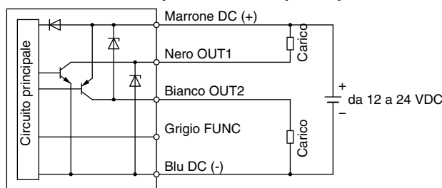
Quando l'uscita è impostata su NPN per il tipo di uscita B
