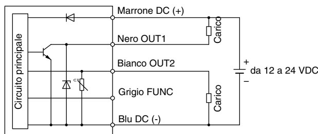
Quando l'uscita è impostata su NPN per il tipo di uscita F
