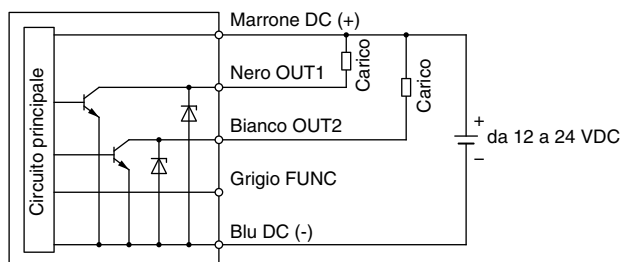
Quando l'uscita è impostata su NPN per il tipo di uscita A
