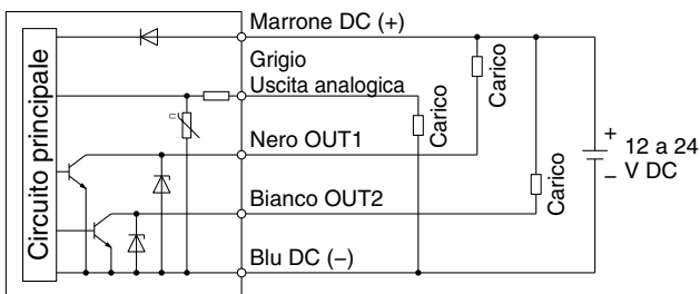
-R: NPN (2 uscite) + Uscita analogica in tensione -S: NPN (2 uscite) + Uscita analogica in corrente
