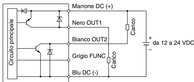
Quando l'uscita è impostata su PNP per il tipo di uscita A
