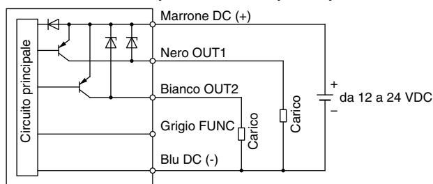
Quando l'uscita è impostata su PNP per il tipo di uscita B
