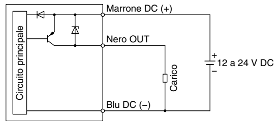
-P PNP (1 uscita)
