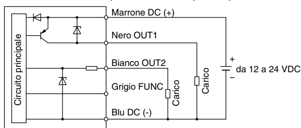
Quando l'uscita è impostata su PNP per il tipo di uscita E
