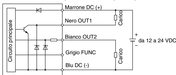
Quando l'uscita è impostata su NPN per il tipo di uscita E
