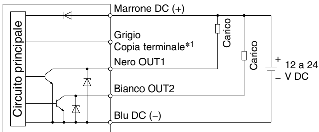
-X NPN (2 uscite) + Funzione di copia
