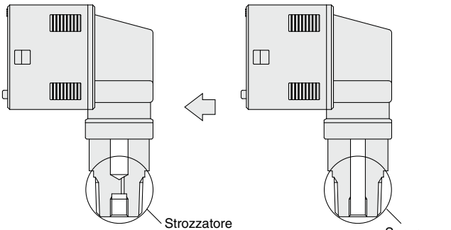
Esecuzioni speciali: "-X510"
