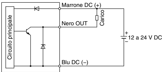
-N NPN (1 uscita)
